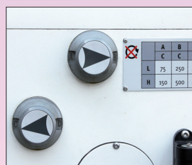
Převodovka DH 28 GS 8 rychlostí, 75 – 2 000 ot/min
