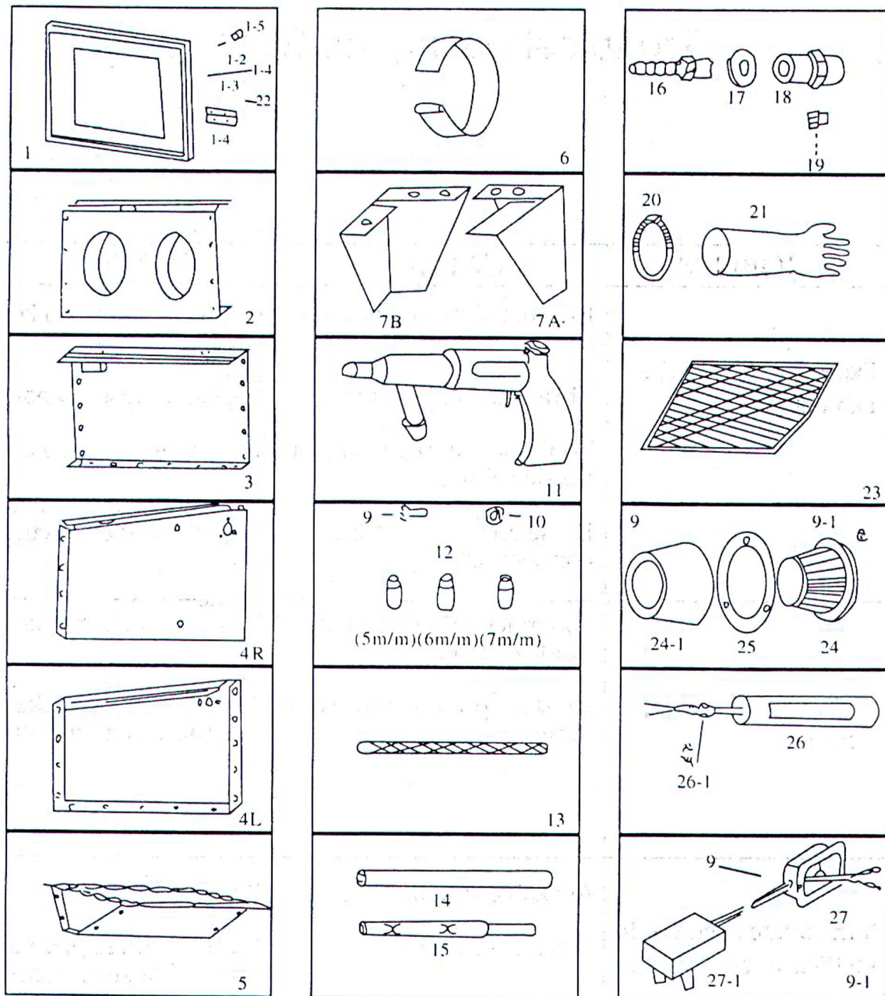
Abb. 7: Rozpadové schéma
